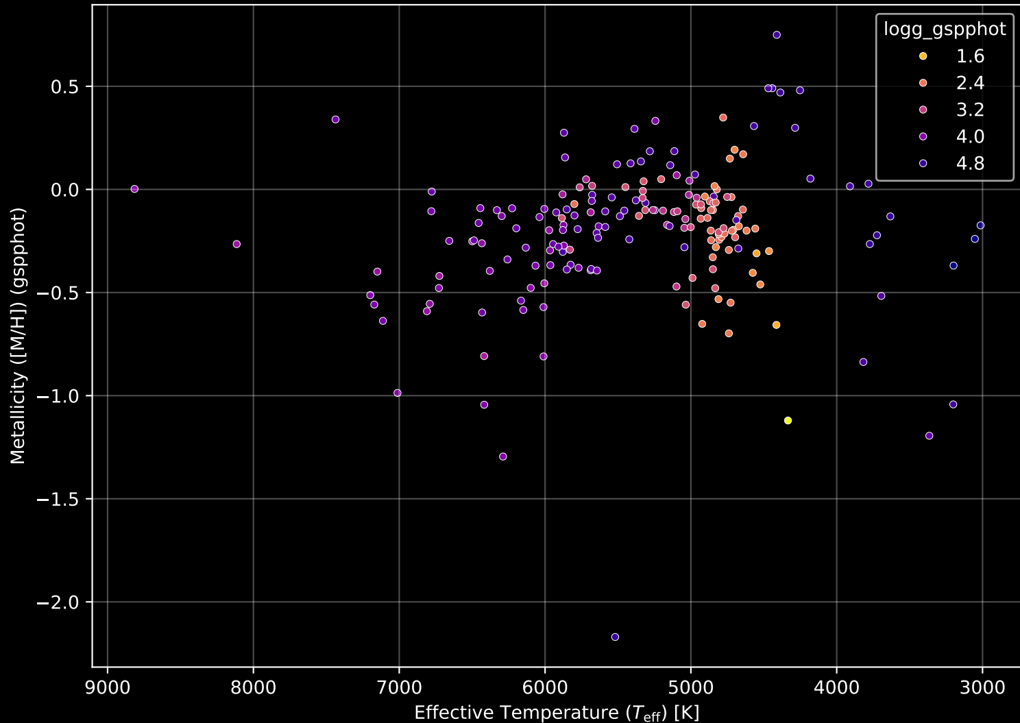
APOGEE DR17 Field: [CVZTILE_105+36_btx] Stellar Population Parameters (n= 191)
